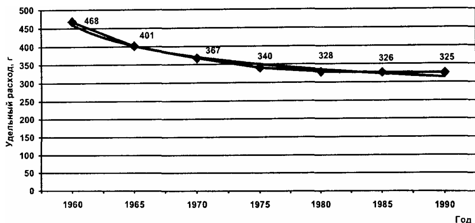
Рис. 4.4. Динамика расхода условного топлива на производство электроэнергии (г на 1 кВт-ч) на электростанциях региона
